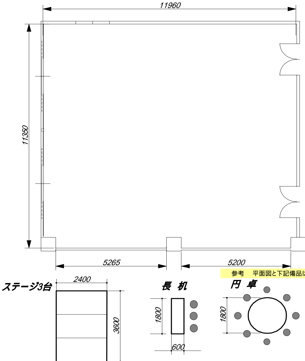
蓬菜 平面図
