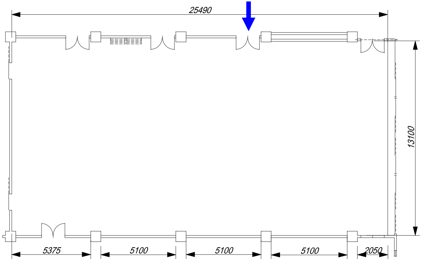
大広間 平面図
