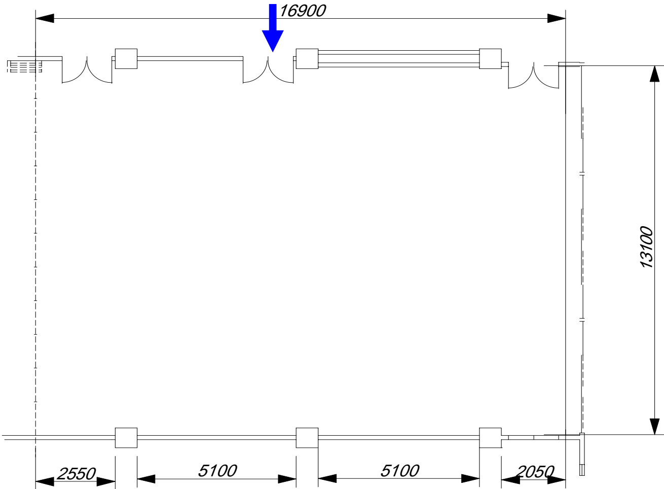
高砂 平面図
